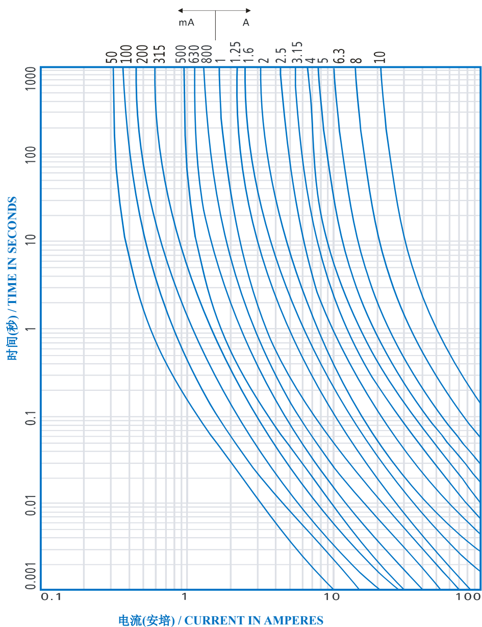
8.5 平均时间电流曲线图 / Average Time Current Curves
